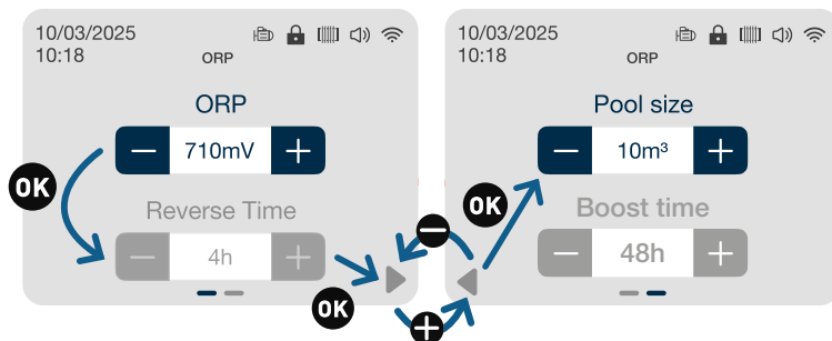
Interface de paramétrage du mode ORP
