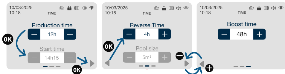
Interfaz de configuración del modo de tiempo
